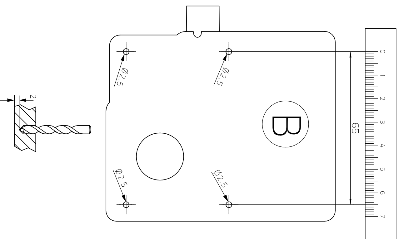
PLANTILLA CERRADURA PUERTA IZQUIERDA TEMPLATE OF LEFT HAND DOOR
