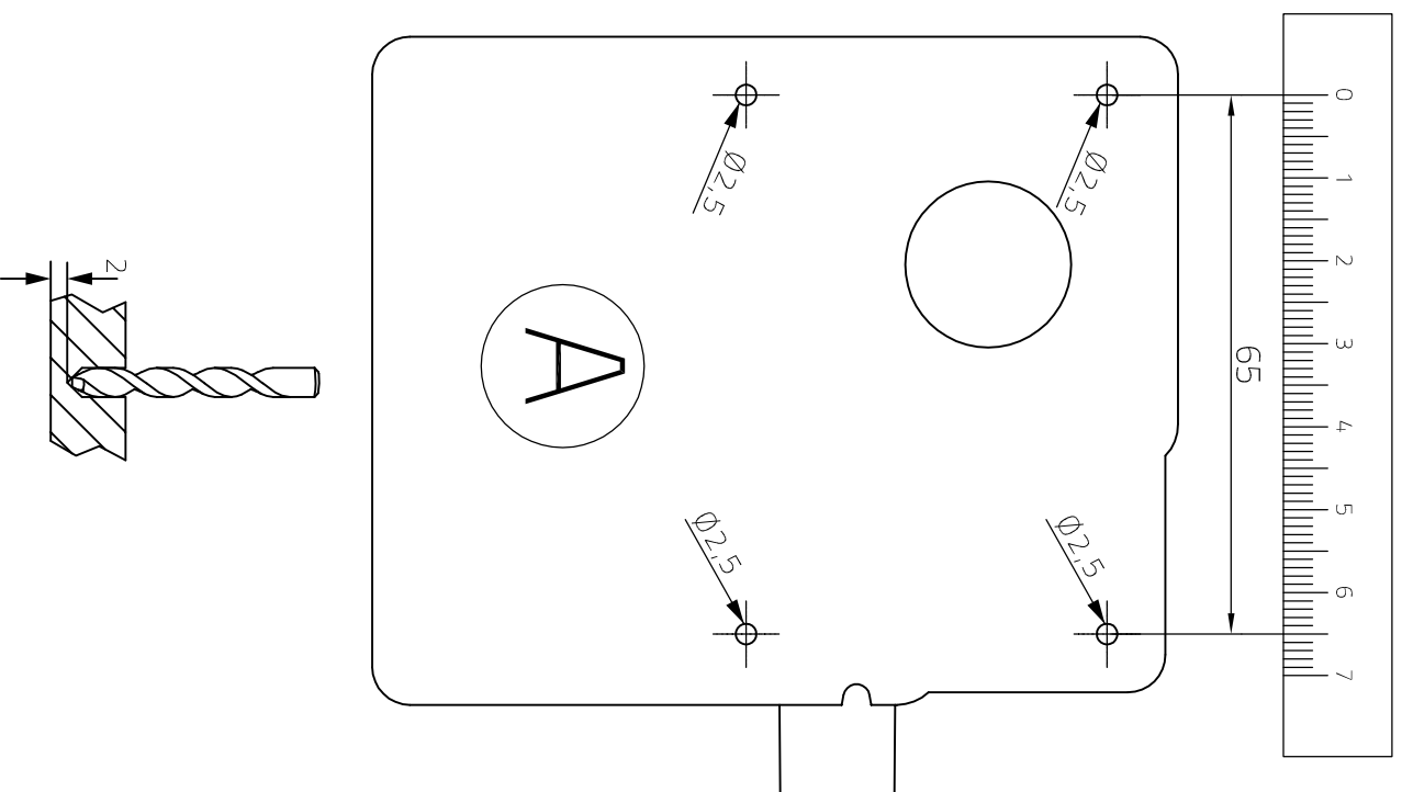
PLANTILLA CERRADURA PUERTA DERECHA TEMPLATE OF RIGHT HAND DOOR
